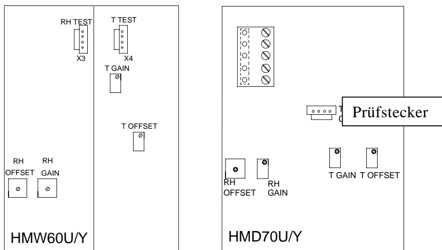
Abbildung 3.3 Kalibrierstecker und Potentiometer bei den Meßwertgebern der HMW60- und der HMW70 - Serie
