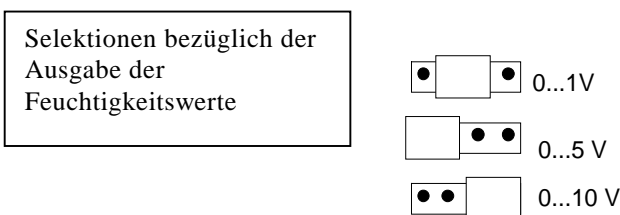
Abbildung 2.3.1 Jumper für den HMD/W70
